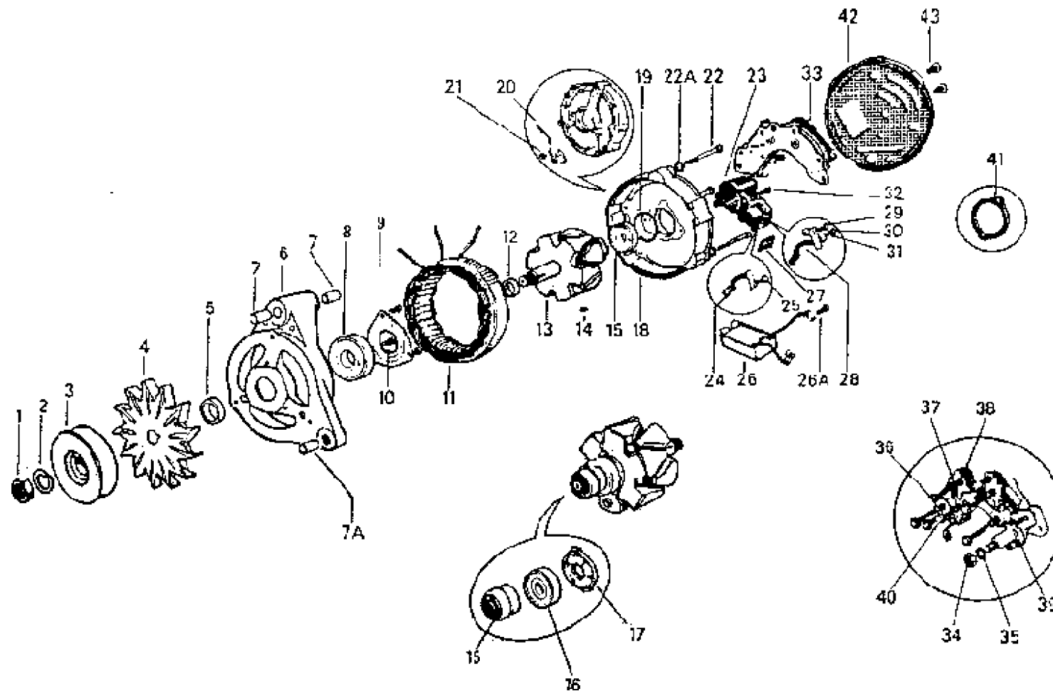
ALTERNATOR (A 115-39)
