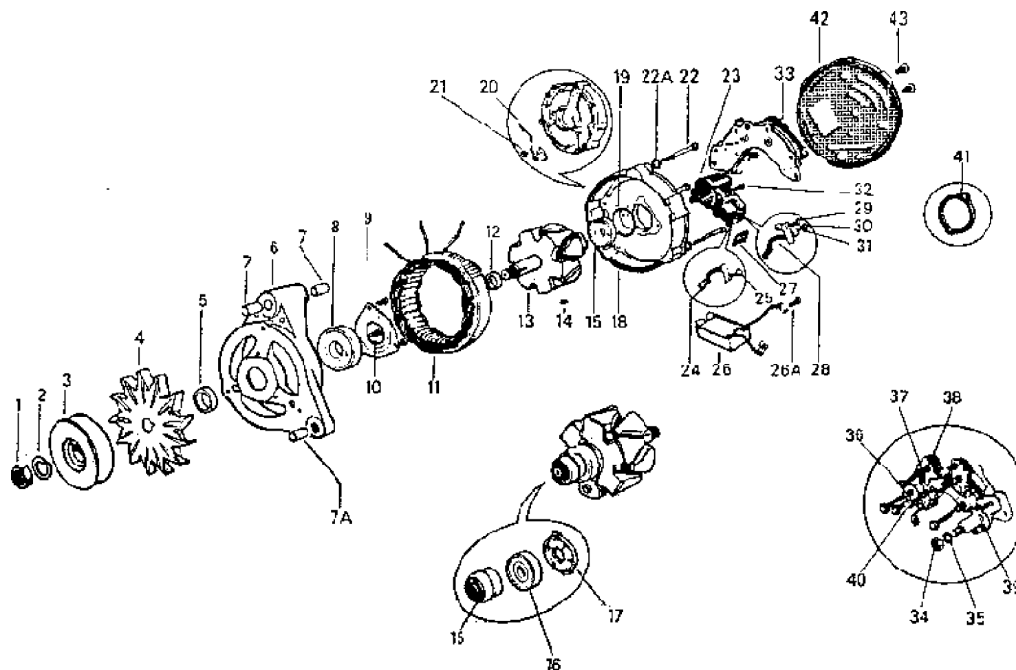
ALTERNATOR (A 115-39)
